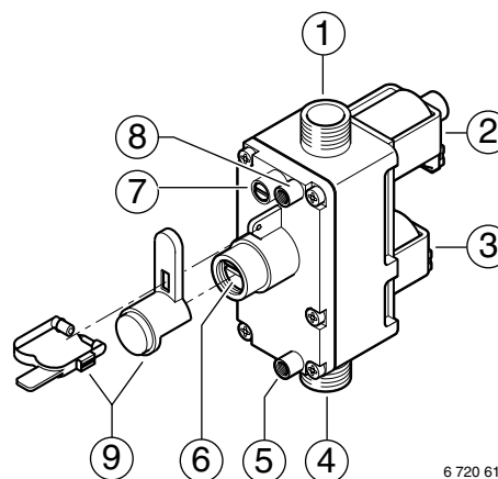
Fig. 26 Cuerpo de gas
