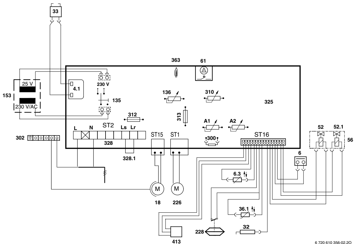
Fig. 2 Cableado eléctrico
