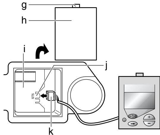
Fig. 20 Tapa falsa
