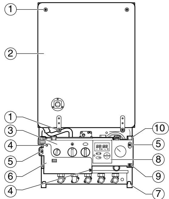
Fig. 40 Sujeción de la cámara de combustión y de la Eurotronic
