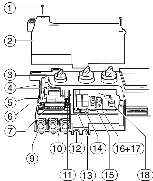
Fig. 13 Conexiones en la Eurotronic
