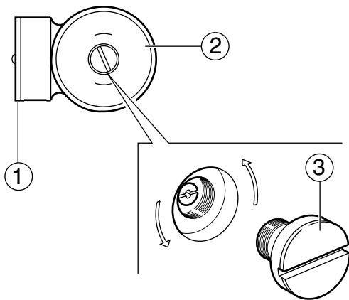
Fig. 23 Purga/desbloqueo de la bomba
