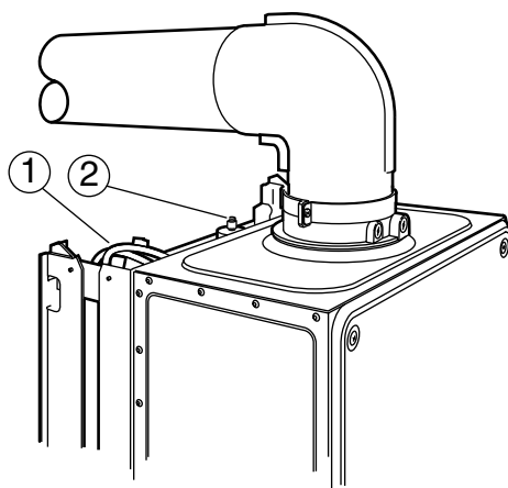
Fig. 22 Purgador automático
