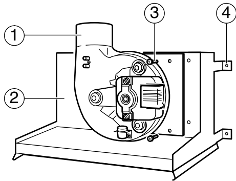
Fig. 43 Ventilador
