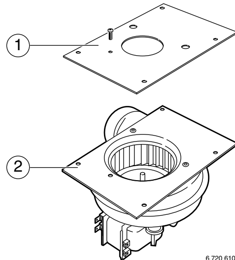
Fig. 45 Ventilador
