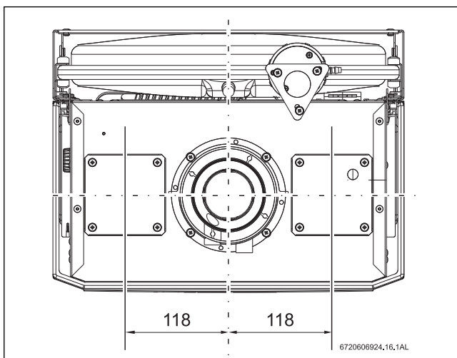
Fig. 2 Vista de topo
