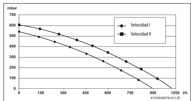
Fig. 35 Curva característica de la bomba
