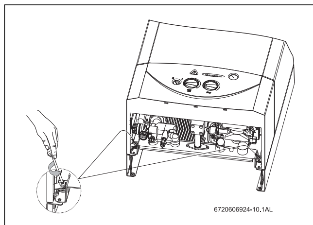
Fig. 7 Parafusos de segurança
