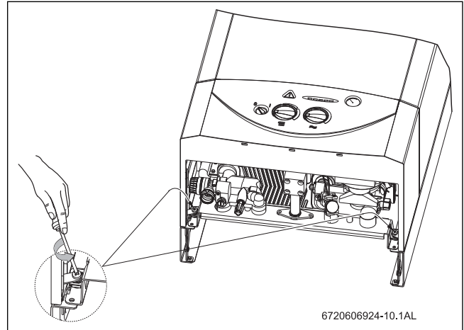
Fig. 37 Tornillos de sujeción
