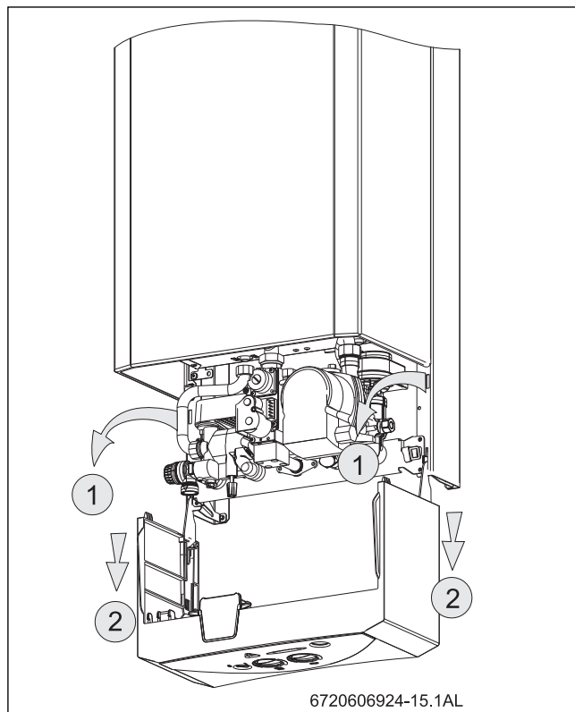
Fig. 26 Posição de serviço para acessibilidade à hidráulica e à electrónica
