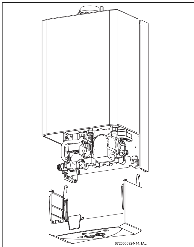
Fig. 39 Desmontaje del panel de mandos
