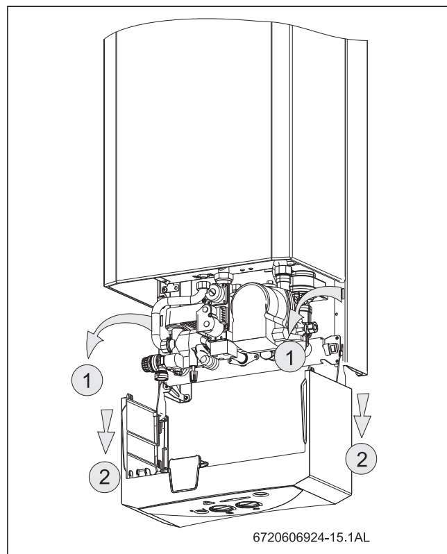
Fig. 55 Posición de servicio para acceso a la parte hidráulica y electrónica
