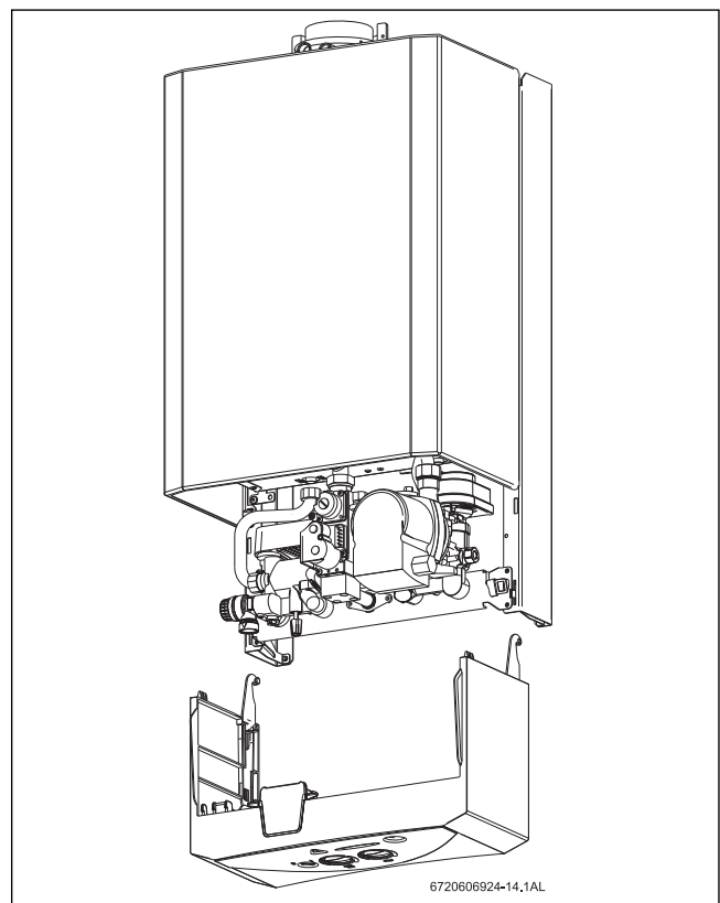
Fig. 9 Retirar painel de comandos
